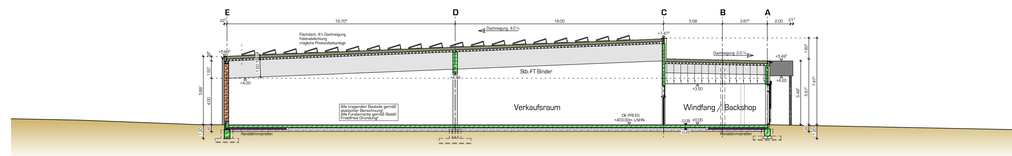
Schnitt A-A
