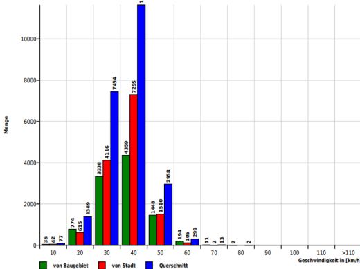
Geschwindigkeits-Histogramm
